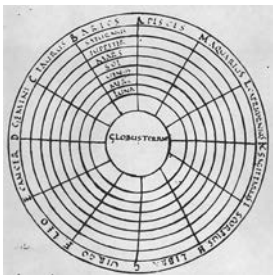
Kuva 1.2 — Planetaariset sfäärit
